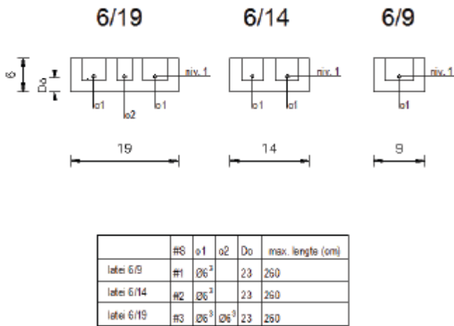
Fig. 2: Configuratie van de beproefde samengestelde lateien
