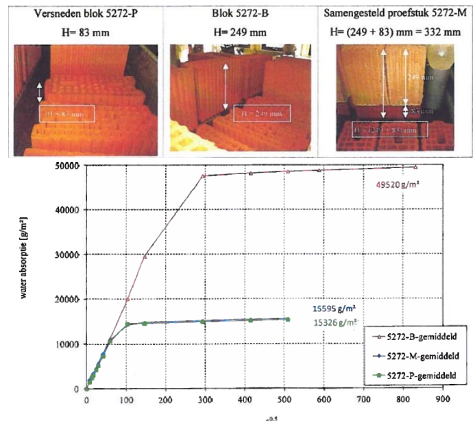
Fig. 3: Wateropslorping door capillariteit opversneden blokken, blokken en samengestelde proefstukken
