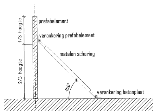
Fig. 4: Plaatsing schoren
