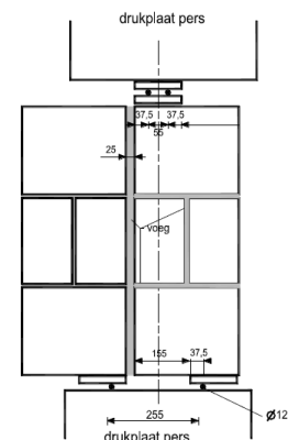
Fig. 7: Proefopstelling afschuivingsproef
