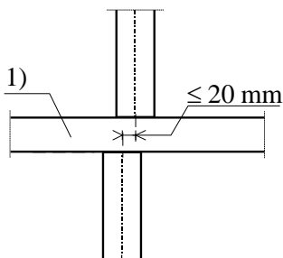
Fig. 5:Toleranties superpositie
